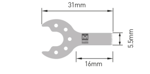
MODEL. HSR-123 Толщина : 0.4mm Ширина : 5.5mm Длина : 16mm
