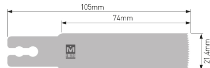
MODEL HCR-151 (Толщина : 0.7mm)
