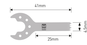
MODEL. HSR-109 Толщина : 0.4mm Ширина : 4.5mm Длина : 25mm
