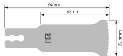
MODEL HCR-150 (Толщина : 0.7mm)
