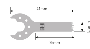
MODEL. HSR-107 Толщина : 0.4mm Ширина : 5.5mm Длина : 25mm
