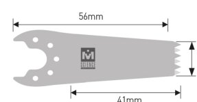
MODEL. HSR-110 Толщина : 0.4mm Ширина : 9.5mm Длина : 41mm
