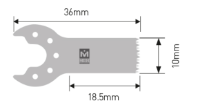
MODEL. HSR-112 Толщина : 0.4mm Ширина : 10mm Длина : 18.5mm
