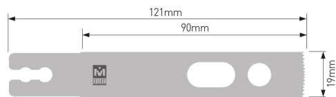
MODEL HCR-102A (Толщина : 1.00mm) MODEL HCR-102B (Толщина : 1.20mm) MODEL HCR-102C (Толщина : 1.27mm) MODEL HCR-102D (Толщина : 1.40mm)
