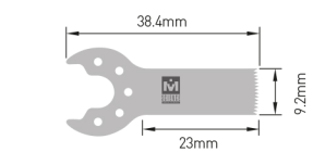
MODEL. HSR-122 Толщина : 0.4mm Ширина : 9.2mm Длина : 23mm
