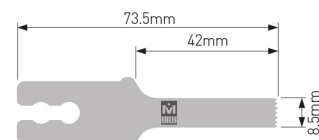
MODEL HCR-156A (Толщина : 0.4mm) MODEL HCR-156B (Толщина : 0.7mm)
