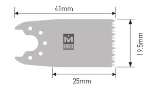
MODEL. HSR-104 Толщина : 0.4mm Ширина : 19.5mm Длина : 25mm
