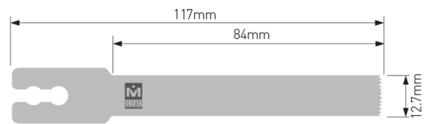
MODEL HCR-103A (Толщина : 1.00mm) MODEL HCR-103B (Толщина : 1.20mm) MODEL HCR-103C (Толщина : 1.27mm) MODEL HCR-103D (Толщина : 1.40mm)
