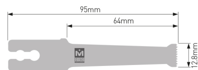
MODEL HCR-153 (Толщина : 0.7mm)
