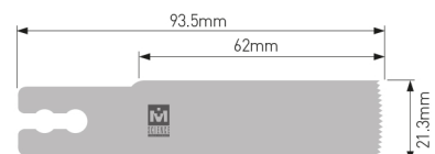
MODEL HCR-152 (Толщина : 0.7mm)
