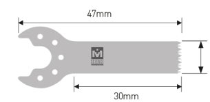
MODEL. HSR-115 Толщина : 0.4mm Ширина : 9.2mm Длина : 30mm
