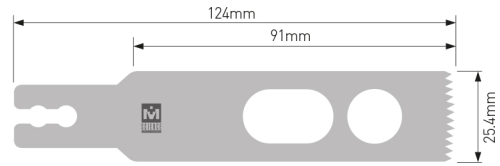
MODEL HCR-100A (Толщина : 1.00mm) MODEL HCR-100B (Толщина : 1.20mm) MODEL HCR-100C (Толщина : 1.27mm) MODEL HCR-100D (Толщина : 1.40mm)
