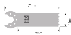
MODEL. HSR-101 Толщина : 0.4mm Ширина : 14mm Длина : 39mm
