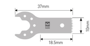
MODEL. HSR-113 Толщина : 0.4mm Ширина : 10mm Длина : 18.5mm
