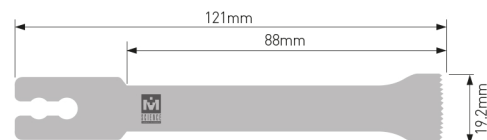
MODEL HCR-105A (Толщина : 1.00mm) MODEL HCR-105B (Толщина : 1.20mm) MODEL HCR-105C (Толщина : 1.27mm) MODEL HCR-105D (Толщина : 1.40mm)
