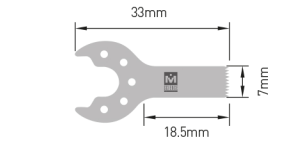
MODEL. HSR-118 Толщина : 0.4mm Ширина : 7mm Длина : 18.5mm
