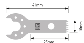
MODEL. HSR-108 Толщина : 0.4mm Ширина : 10mm Длина : 25mm
