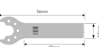
MODEL. HSR-116 Толщина : 0.4mm Ширина : 9.5mm Длина : 39mm
