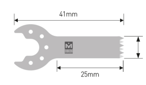
MODEL. HSR-106 Толщина : 0.4mm Ширина : 8.4mm Длина : 25mm
