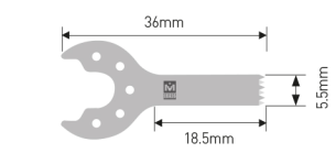
MODEL. HSR-111 Толщина : 0.4mm Ширина : 5.5mm Длина : 18.5mm
