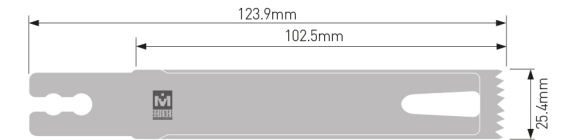
MODEL HCR-100HB (Толщина : 1.20mm) MODEL HCR-100HC (Толщина : 1.27mm) MODEL HCR-100HD (Толщина : 1.40mm)
