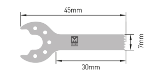
MODEL. HSR-117 Толщина : 0.4mm Ширина : 7mm Длина : 30mm
