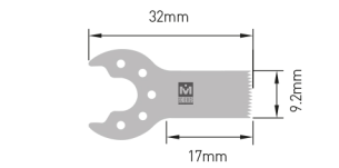
MODEL. HSR-119 Толщина : 0.4mm Ширина : 9.2mm Длина : 17mm
