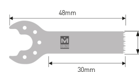
MODEL. HSR-114 Толщина : 0.4mm Ширина : 9mm Длина : 30mm
