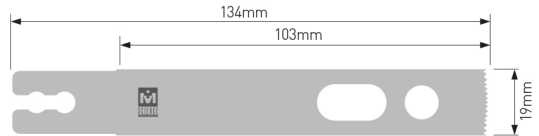
MODEL HCR-101A (Толщина : 1.00mm) MODEL HCR-101B (Толщина : 1.20mm) MODEL HCR-101C (Толщина : 1.27mm) MODEL HCR-101D (Толщина : 1.40mm)
