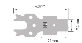
MODEL. HSR-120 Толщина : 0.4mm Ширина : 9.4mm Длина : 21mm
